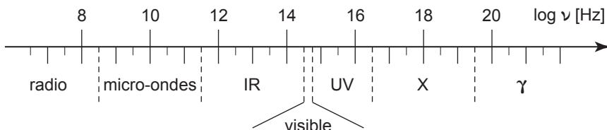
Figure 1.1 - Les différentes gammes du rayonnement électromagnétique
